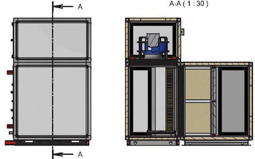
A-A (1 : 30)
